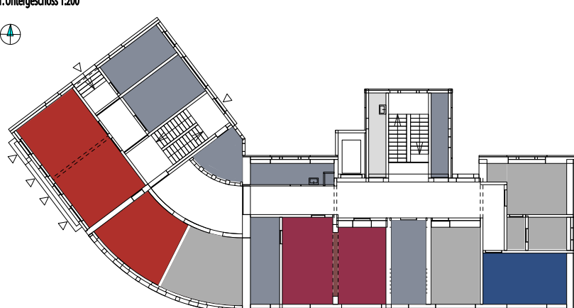
1.Untergeschoss 1:200
