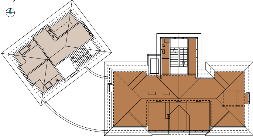
Dachgeschoss 1:200
